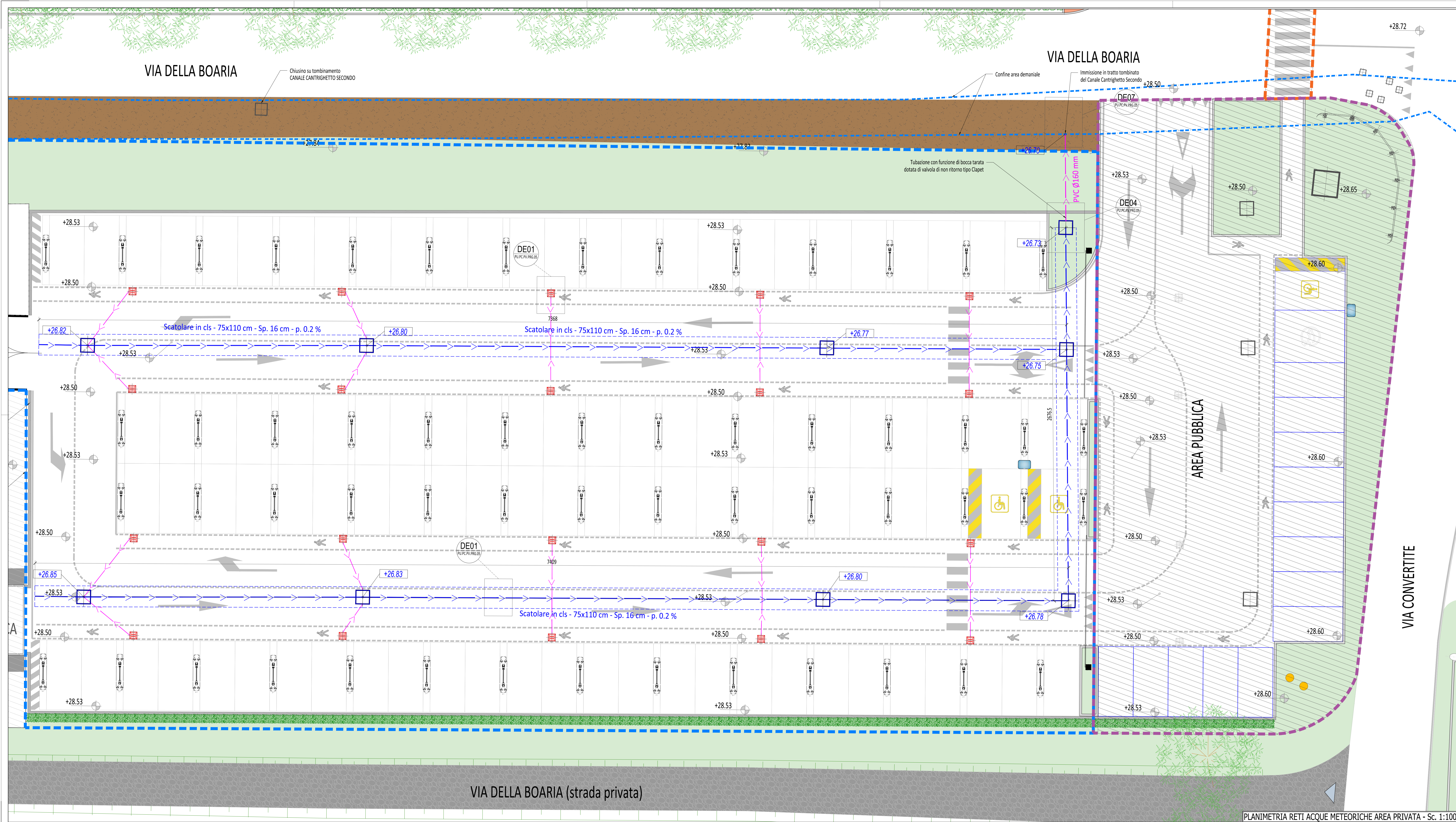
PLANIMETRIA RETI ACQUE METEORICHE AREA PRIVATA - Sc. 1:100
